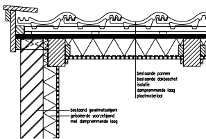
tussen de sporen isoleren
