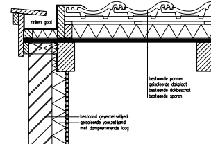
op sporen isoleren met verholven goot
