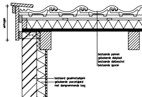
op sporen isoleren met verhoogde windveer
