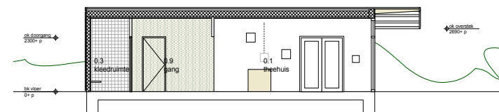
Doorsnede B-B
