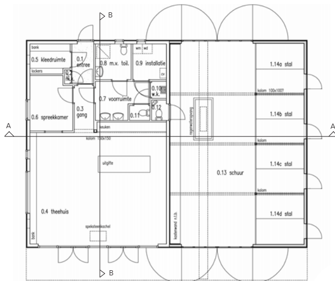
Begane grond
