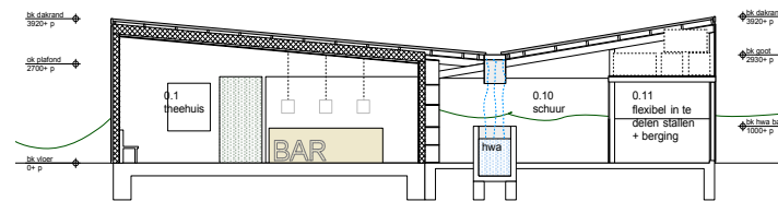
Doorsnede A-A
